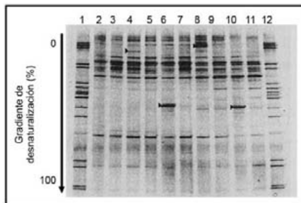
Figura 3. Gel de DNA en gradiente de desnaturalización (DGGE). Los carriles 1 y 12 muestran al marcador de especies bacterianas; del carril 2 al 11 son las muestras de pacientes. La identidad inicial se establece por la movilidad con respecto al marcador de especies. 35
