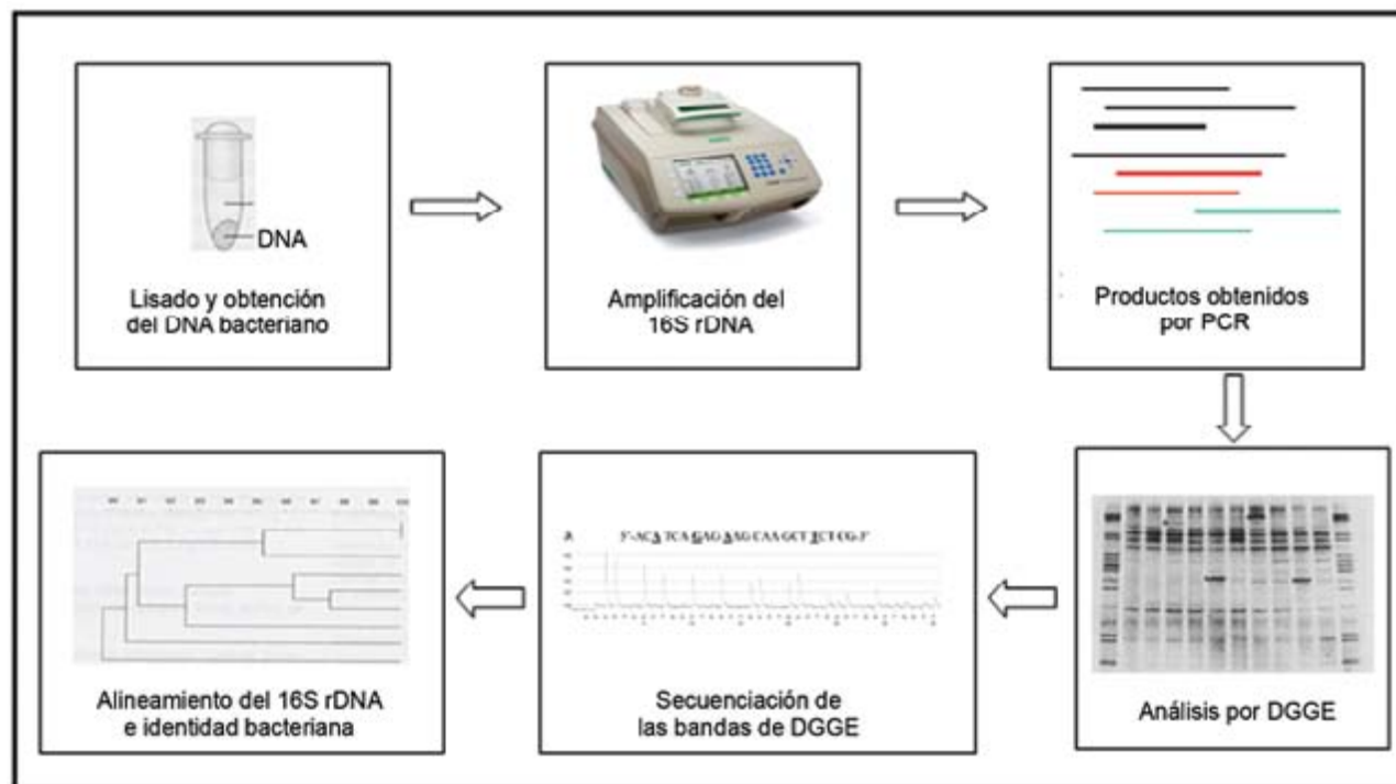
Figura 4. Diagrama de flujo para identificar a las bacterias mediante la PCR-DGGE. La identificación inicial de las bacterias se determina por la movilidad de los diferentes productos de PCR con respecto al marcador de referencia. La identidad bacteriana se realiza por el alineamiento con el banco de genes y permite predecir la relación filogenética hasta del 100%.
