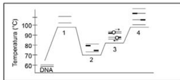
Figura 1. Amplificación del DNA por la PCR. El DNA de interés es desnaturalizado permitiendo la separación de la doble cadena (1); la disminución de la temperatura, permite que el iniciador de alineamiento y se dé la unión a regiones específicas del DNA (2); un segundo incremento de la temperatura activa a la polimerasa y comienza la extensión de la cadena de DNA, mediante la incorporación de los nucleótidos de adenina, citosina, timina y guanina (3). El ciclo inicia nuevamente (4). La amplificación de DNA es exponencial con respecto a la concentración inicial.
