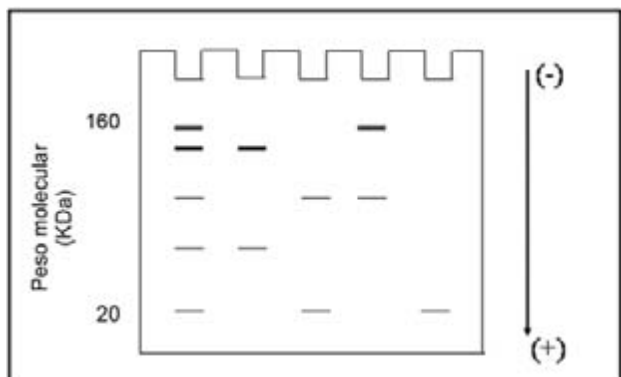
Figura 2. Migración diferencial de las biomoléculas contenidas en una muestra. La carga eléctrica va de arriba (-) hacia abajo (+). El peso molecular es en unidades de kilo daltones (kDa) que equivalen al peso aproximado del átomo de hidrógeno.
