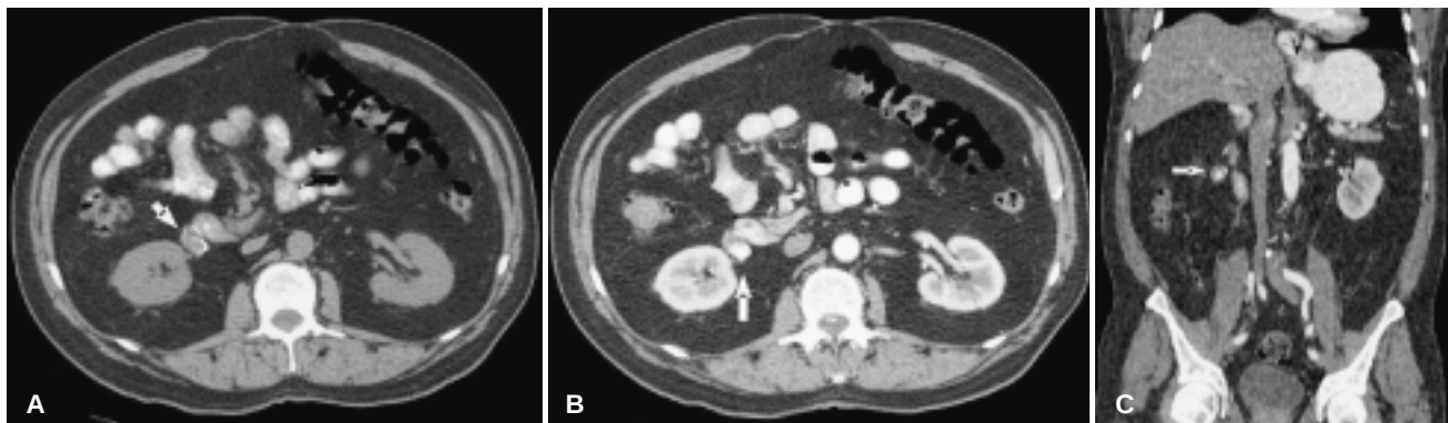
Figura 10. (A, B y C). Caso 4. Cortes axiales de TC en fase simple y fase arterial ( A y B , respectivamente) en donde se identifica imagen sacular en topografía parahiliar renal derecha, asociada a calcificaciones lineares; posterior al medio de contraste hay reforzamiento intraluminal, lo que permite delimitar la presencia del trombo parietal (flechas), C) RMP en plano coronal, fase arterial, que permite delimitar el trombo periférico al reforzamiento de la luz intravascular (flecha).
