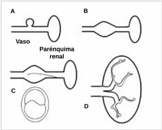
Figura 3. A) Aneurisma sacular, B) aneurisma fusiforme, C) aneurisma disecante y su vista en un corte axial a través del aneurisma (abajo) y D) aneurisma intrarrenal.
