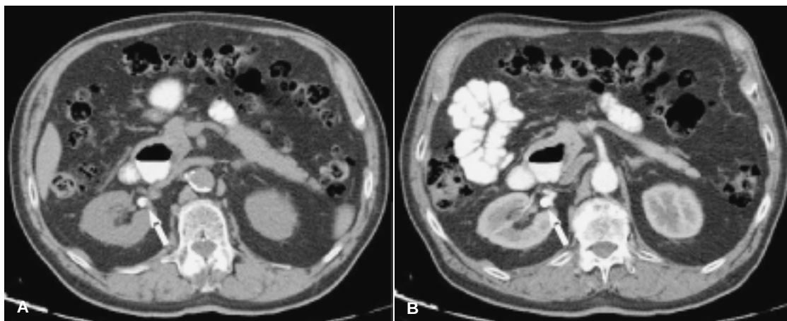
Figura 8. (A y B) Caso 2. Cortes axiales de TC en fase simple (A) y fase arterial (B) donde se observa calcificación redonda puntiforme en topografía hiliar derecha, que presenta reforzamiento con el medio de contraste (flechas).
