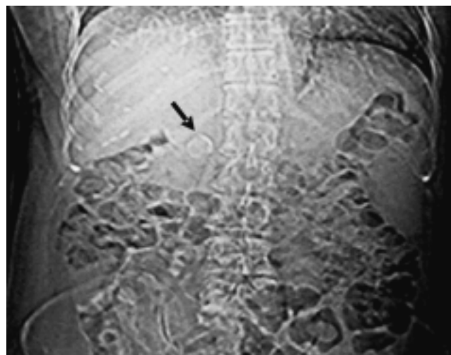
Figura 5. Caso 6. Topograma que muestra imagen de densidad cálcica, en anillo, proyectada en el hipocondrio derecho (flecha negra).
