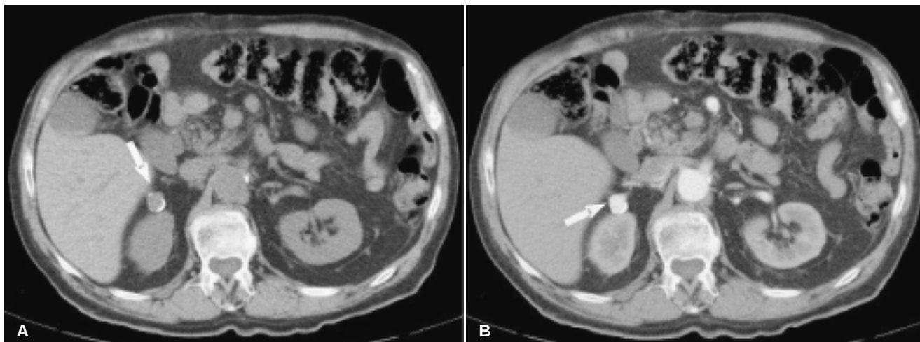
Figura 9. (A y B) Caso 5. Cortes axiales de TC en fase simple y fase arterial, respectivamente, donde se identifica imagen sacular parahiliar renal derecha, con una calcificación parietal en forma de cuña que presentó reforzamiento intraluminal posterior al medio de contraste (flechas).
