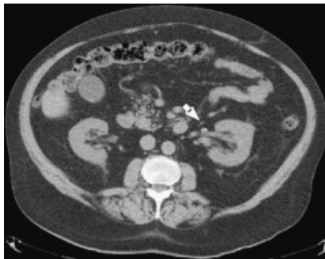
Figura 7. Caso 3. Corte axial de TC en fase simple donde se observa imagen sacular asociada a calcificación puntiforme en la pared de la arteria renal izquierda (flecha).
