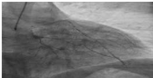
Figura T2-1: Angiografía coronaria izquierda, proyección OAD caudal al octavo latido de la inyección.
