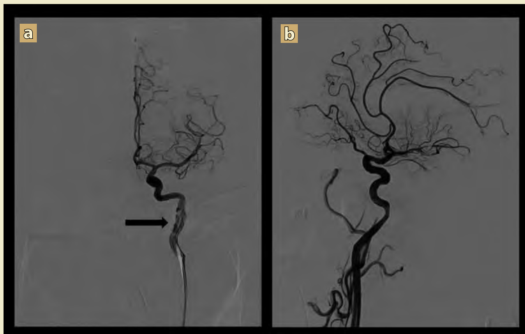
Figura 4. Procedimiento endovascular
