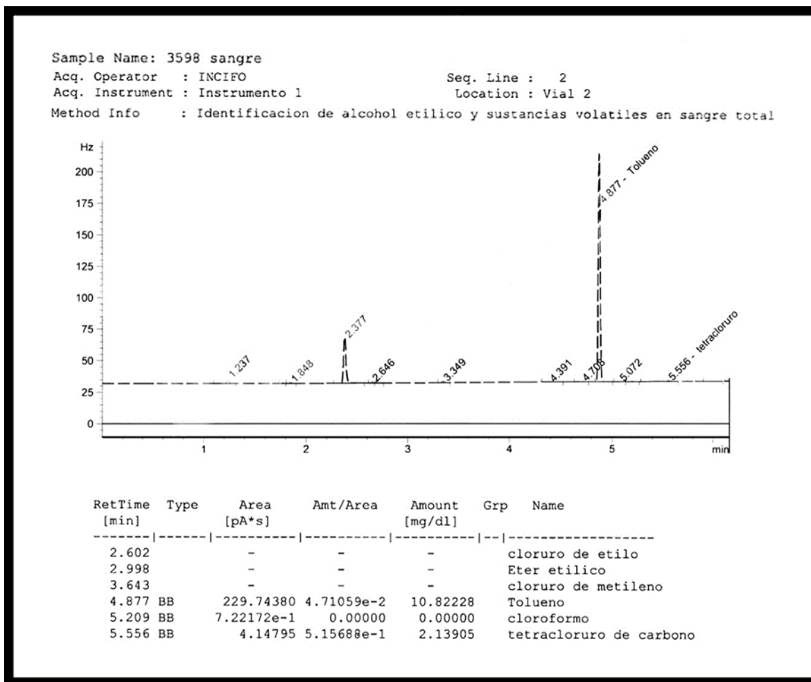
FIGURA 1. Cromatograma de la muestra sanguínea, la cual fue positiva para tolueno. Analizada por cromatografía de gases con head space.
