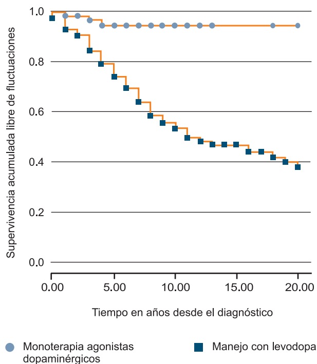
Figura 1 Curva de Kaplan-Meier al comparar los grupos de monoterapia con agonista dopaminérgico y con levodopa (monoterapia o politerapia). Log-rank < 0.001 . Supervivencia expresada como años libres de fluctuaciones
