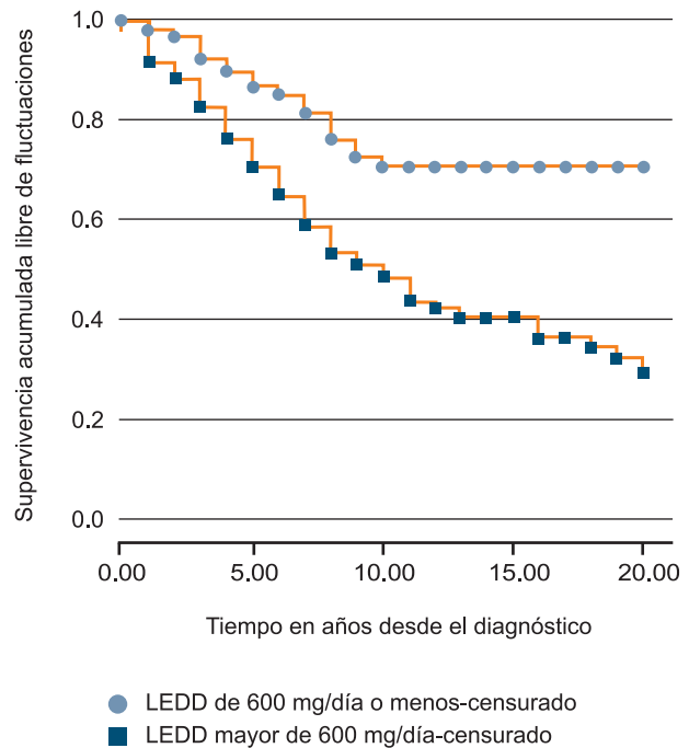
Figura 2 Curva de Kaplan-Meier al comparar los grupos con dosis diaria de levodopa menor de 600 mg y \geq 600 mg. Log-rank < 0.001. Supervivencia expresada como años libres de fluctuaciones
