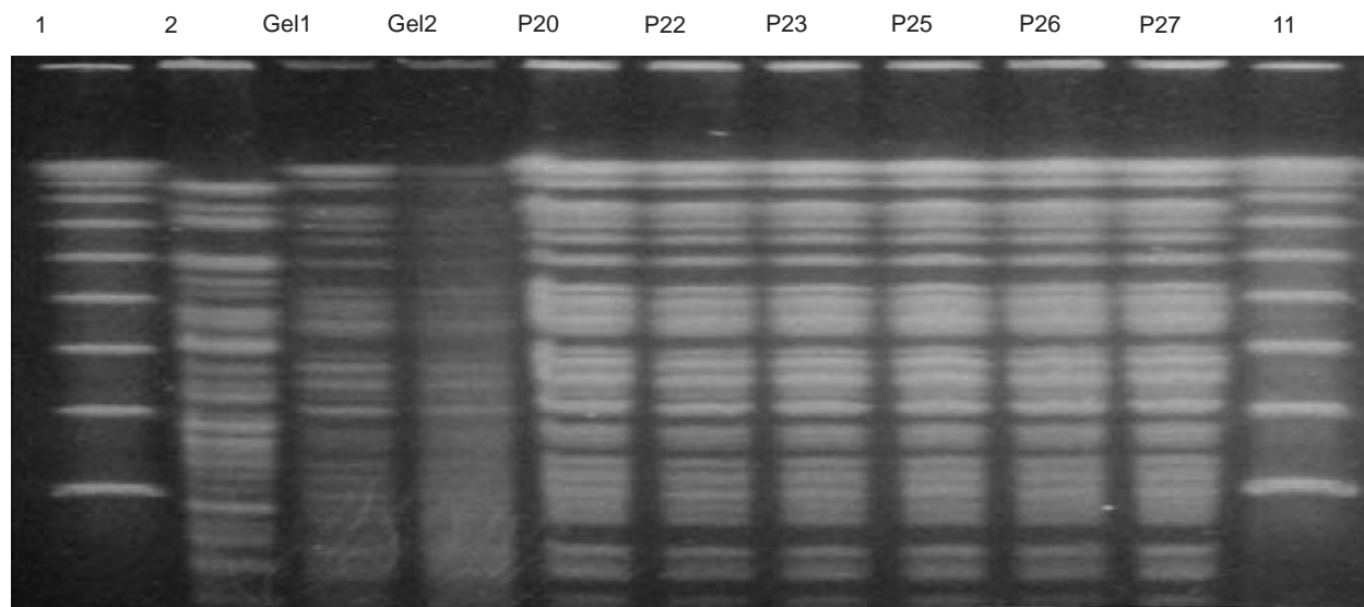
Figura 1 | Electroforesis por campos pulsados de B. cepacia . Carriles 1 y 11: marcadores lambda ladder de peso molecular. Carril 2: cepa no relacionada. Carriles Gel1 y Gel2: cepas aisladas de dos envases del gel lubricante contaminado. Carriles P20 a P27: cepas aisladas de urocultivos de pacientes con infección de vías urinarias asociada con catéter. (Las cepas de los casos 1 a 19 no pudieron ser recuperadas)
