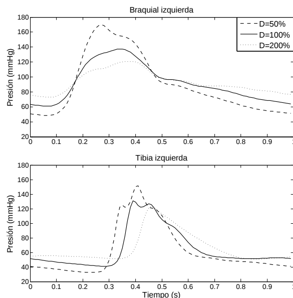
Figura 3: Formas de onda de presión en las arterias braquial y tibia anterior, para tres niveles de distensibilidad ( D ) alterada en todos los segmentos excepto en los segmentos braquiales y tibias.
