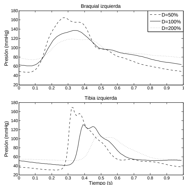
Figura 2. Formas de onda de presión en las arterias braquial y tibia anterior, para tres niveles de distensibilidad ( D ) alterada en todos los segmentos.
