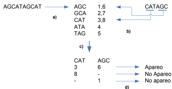
Figura 5. El algoritmo de hash. a) El genoma se divide en 3 –mers traslapados y la posición de cada uno de estos se almacena en la tabla. b) La lectura también se divide en semillas de tamaño 3 y se buscan en la tabla Hash. c) Las posiciones para cada semilla se comparan unas con otras c) Si se obtienen las posiciones adjuntas y en el orden correcto, estas representan una alineación exacta.
