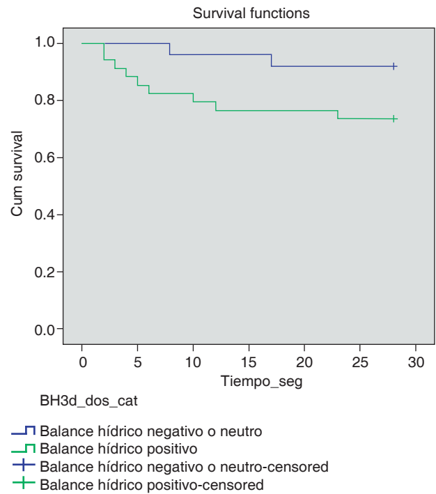
Figura 2. Curva de Kaplan-Meier para la diferencia en la supervivencia entre el grupo de balance hídrico positivo y negativo al tercer día de estancia en la UCI.
