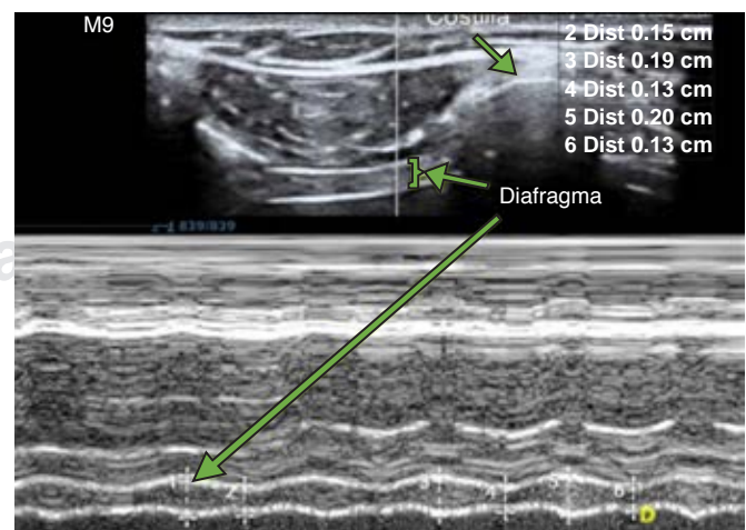
Figura 2: Imagen ultrasonográfica en la que se observa (flecha verde) el grosor diafragmático en modo 2D (superior) y modo M (inferior).
