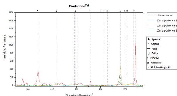
Figura 2. Espectros Raman Biodentine™.
