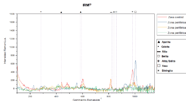
Figura 5. Espectros Raman control negativo IRM®.
