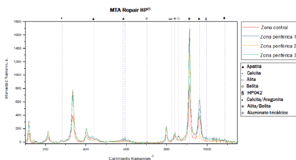
Figura 3. Espectros Raman MTA Repair HP®.
