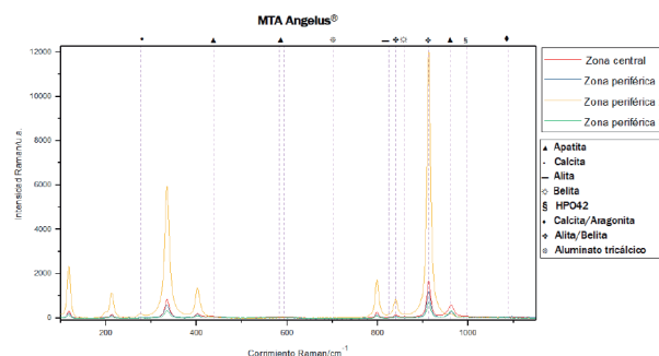
Figura 4. Espectros Raman control positivo MTA Angelus®.
