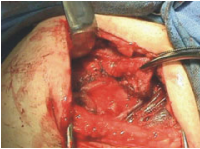
Figura 3. Reparación subescapular.
