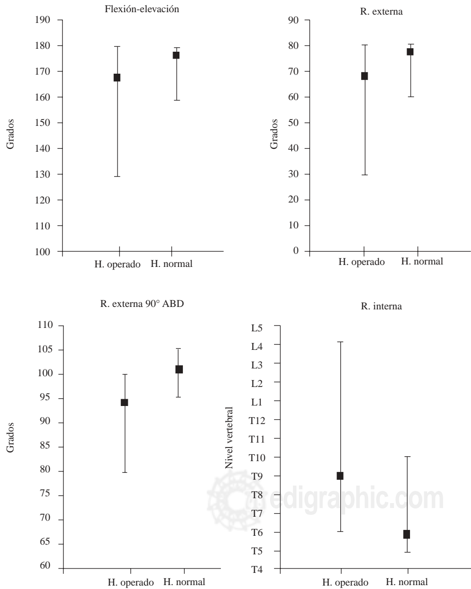
Figura 3. Reparación subescapular.
