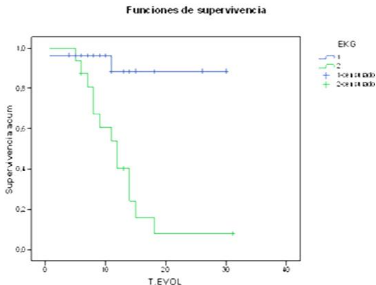
Figura 1. Supervivencia y arritmias en el EKG.
