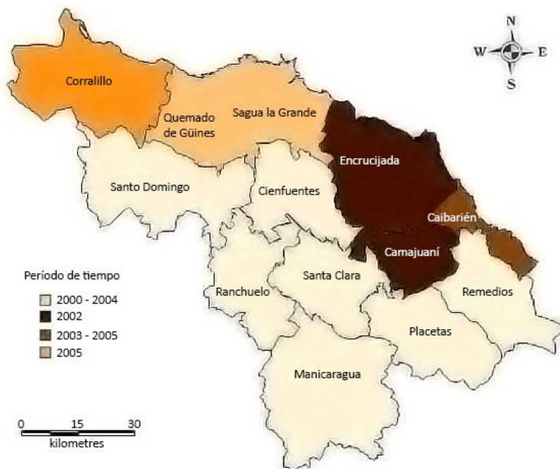
Fig. 1 -Conglomerados puramente espaciales de la incidencia de leucemia aguda en niños. Villa Clara 2000-2012.
