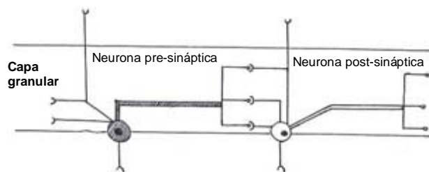
Fig. 4. Conexión entre dos interneuronas en canasta. La transmisión sináptica en estas sinapsis se verá deprimida tanto después de la aplicación de pulsos pareados de estimulación (PPD; pre-sináptica) como después de la aplicación de pulsos múltiples repetidos de estimulación (MRPD; post-sináptica). Asimismo, el tiempo de duración de la inhibición entre interneuronas será más rápido que aquel entre interneuronas y neuronas granulosas, lo que afectará la actividad mnemónica normal.
