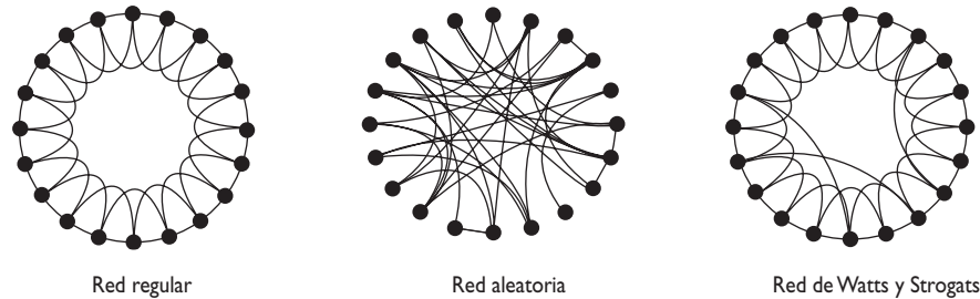
FIGURA 3. REDES COMPLEJAS
