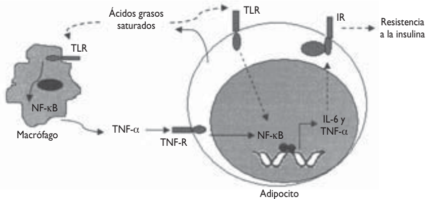
FIGURA 1. EFECTO DE LOS ÁCIDOS GRASOS SATURADOS EN EL ADIPOCITO Y EN EL MACRÓFAGO. DURANTE LA INFILTRACIÓN DE LOS MACRÓFAGOS AL TEJIDO ADIPOSITO SE PRODUCE UN AUMENTO EN LA SECRECIÓN DEL TNF-α; ESTE FACTOR ACTIVA TANTO A LA LIPÓLISIS COMO AL NF-κB A TRAVÉS DE SU RECEPTOR (TNF-R) QUE SE ENCUENTRA EN EL ADIPOCITO. POR OTRO LADO, LOS ÁCIDOS GRASOS SATURADOS, PRODUCIDOS POR EL ADIPOCITO, ESTÁN INVOLUCRADOS EN LA ACTIVACIÓN DE LOS TLRs EN EL MACRÓFAGO Y EN EL PROPIO ADIPOCITO; ESTOS RECEPTORES TAMBIÉN FAVORECE LA ACTIVACIÓN DEL NF-κB, LO CUAL CONTRIBUYE A INCREMENTAR LA SECRECIÓN DE CITOCINAS INFLAMATORIAS EN ESTAS DOS ESTIRPES CELULARES. COMO CONSECUENCIA DISMINUYE LA ACTIVACIÓN DEL SUSTRATO DEL RECEPTOR DE INSULINA (IRS), CAUSANDO RESISTENCIA A LA INSULINA EN EL ADIPOCITO
